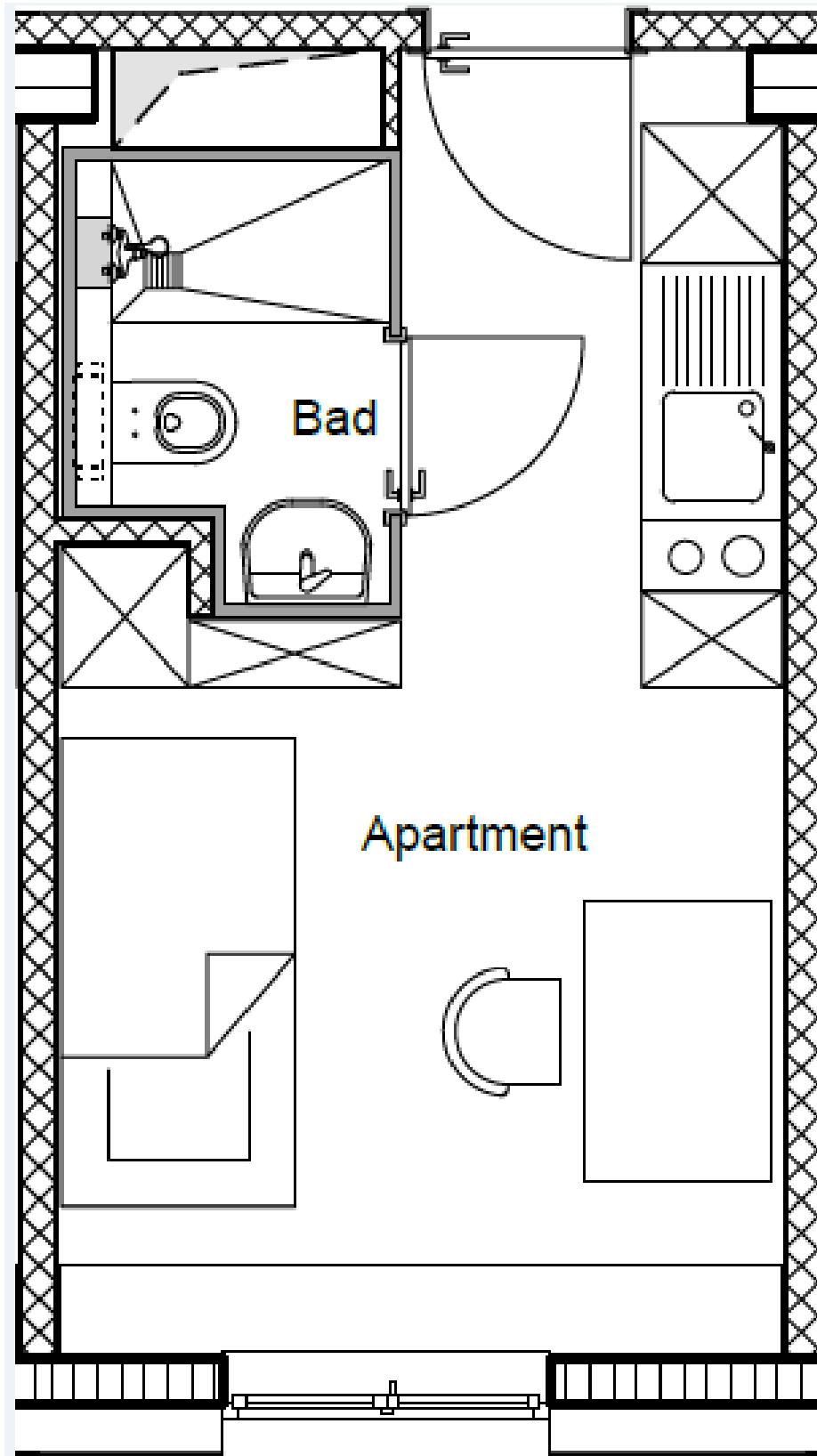
Grundriss Einzelapartment ca. 15,92 m 2 - Selma-Lagerlöf-Str. 10-16, 13189 Berlin Pankow
