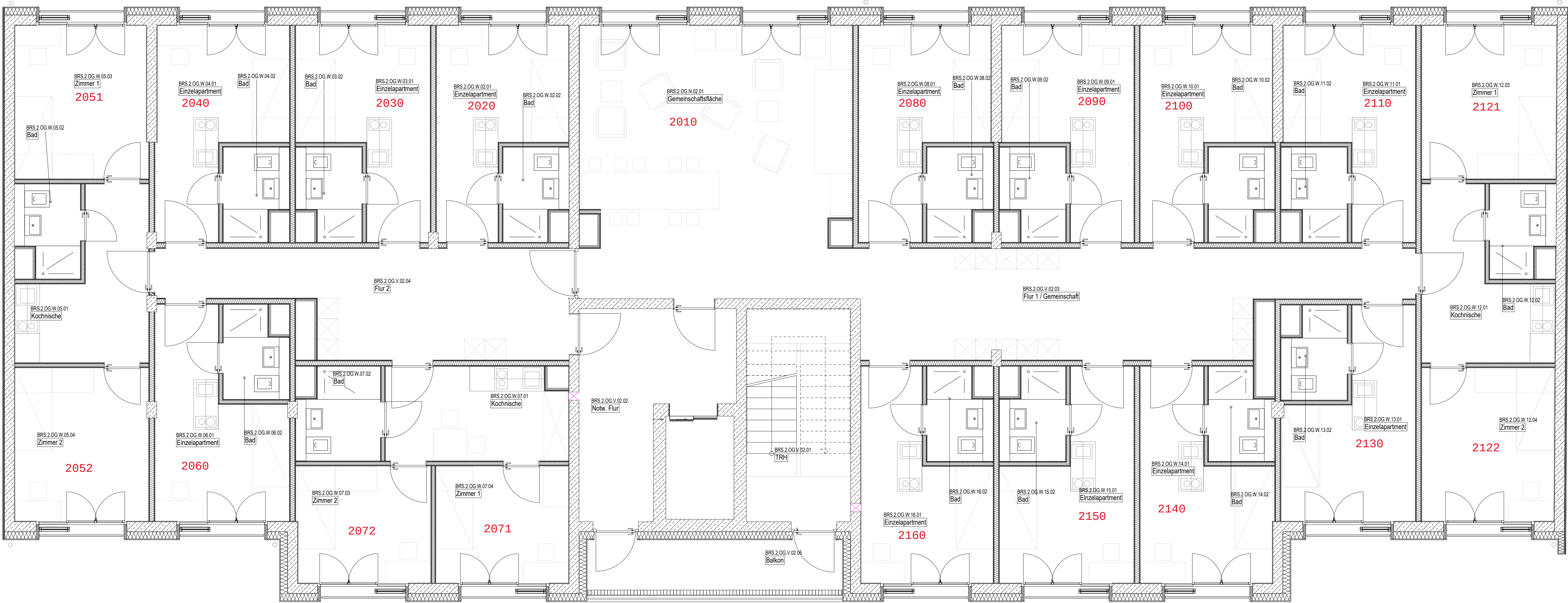
2. OBERGESCHOSS
